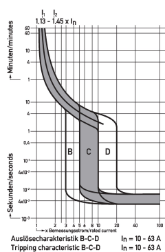
Diagramme Leitungsschutzschalter DLS 6i D40-3
