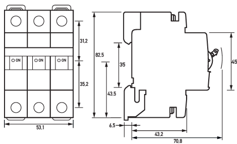
Maßzeichnung Leitungsschutzschalter DLS 6i D40-3
